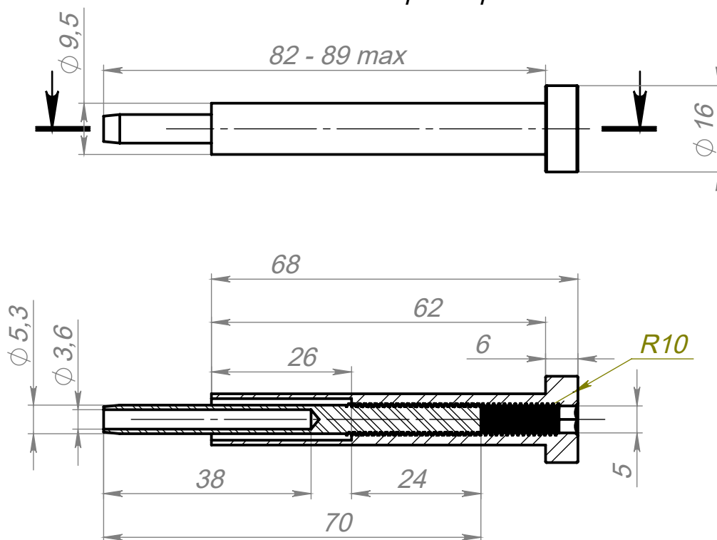
Основные размеры
